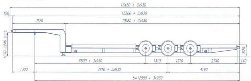
VERSIONE 3S3602
